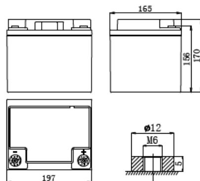
Вывод В-М6
